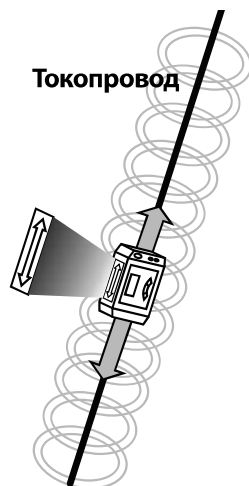
Рис. 15 – Расположение относительно трассы – индукционный режим
