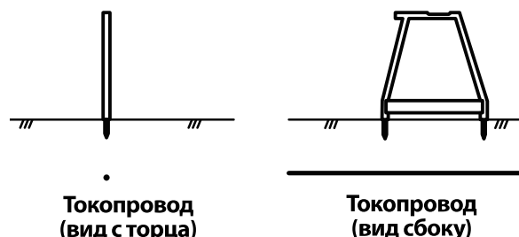
Рис. 10 – Расположение приемника
