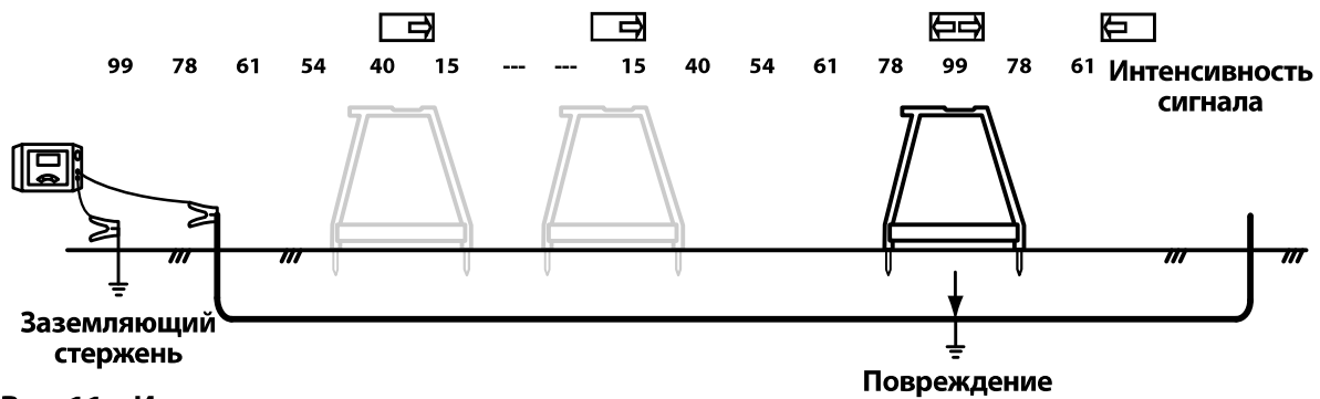
Рис. 11 – Интенсивность сигнала
