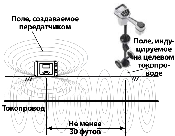
Рис. 16 – Расположение относительно трассы – индукционный режим
