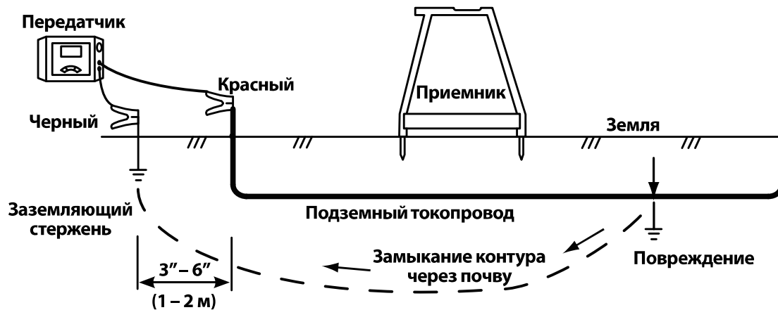
Рис. 8 – Соединения передатчика для поиска повреждения
